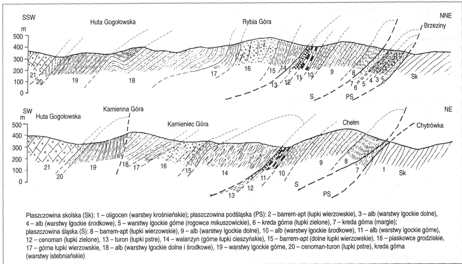
Przekroje geologiczne przez brzeżną strefę płazczowiny śląskiej (wg F. Szymakowskiej — niepublikowane)
