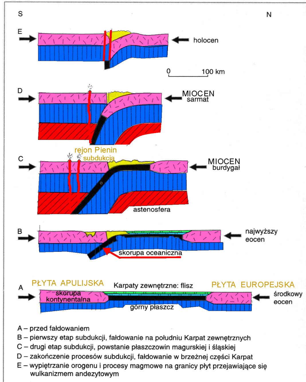
Geneza Karpat zewnętrznych (interpretacja wg A.K. Tokarskiego, 1978 — zmodyfikowana)
