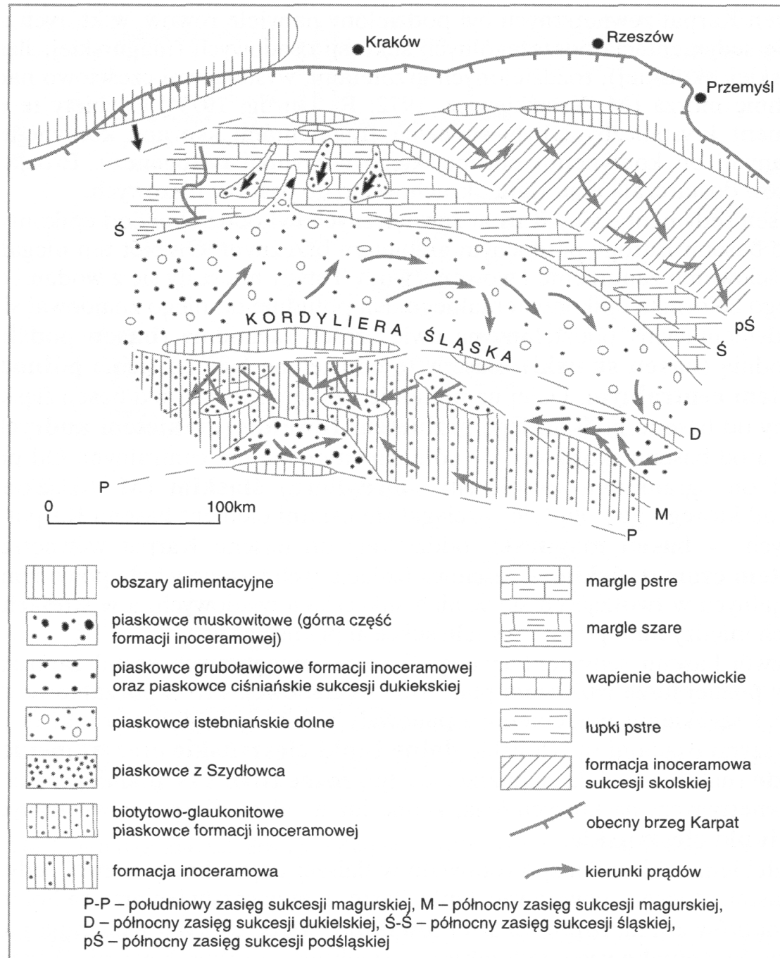
Paleogeografia polskiej części Karpat zewnętrznych w późnej kredzie
