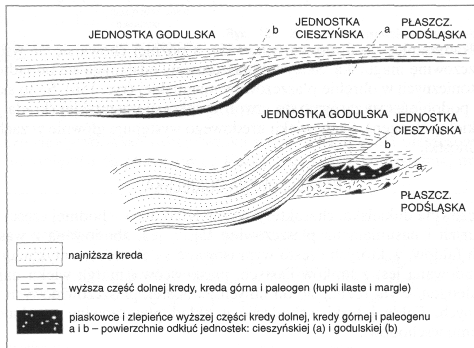
Powstanie jednostki cieszyńskiej i godulskiej w obrębie zachodniej części płaszczowiny śląskiej (wg M. Książkiewicza, 1972)
