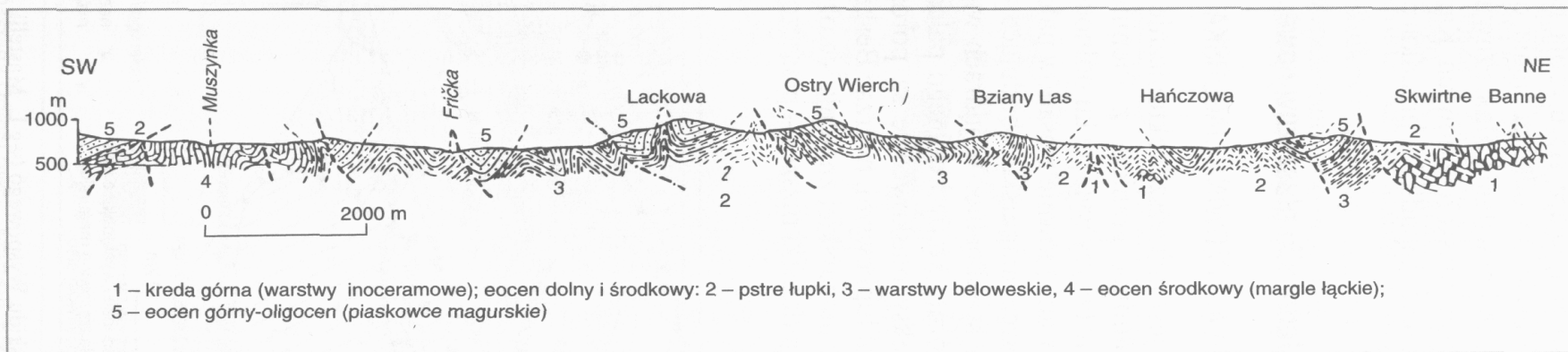
Przekrój przez płaszczwinę magurską między Hańczową a Tyliczem (wg S. Węclawika, 1969)
