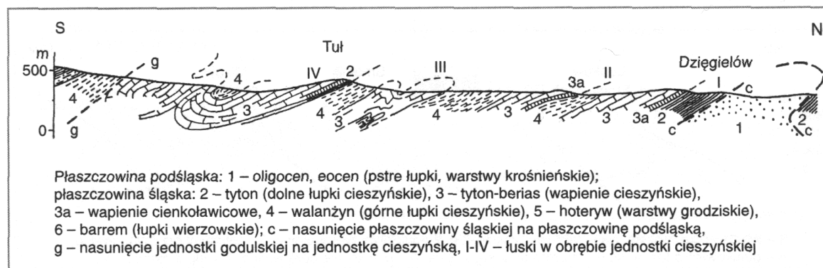
Przekrój geologiczny przez jednostkę cieszyńską między Olzą a Wisłą (wg M. Książkiewicza, 1972)
