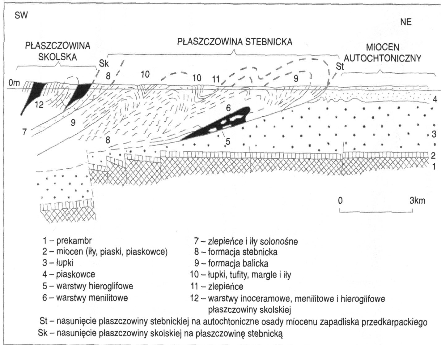
Przekrój geologiczny przez płaszczowinę stebnicką na południe od Przemyśla
