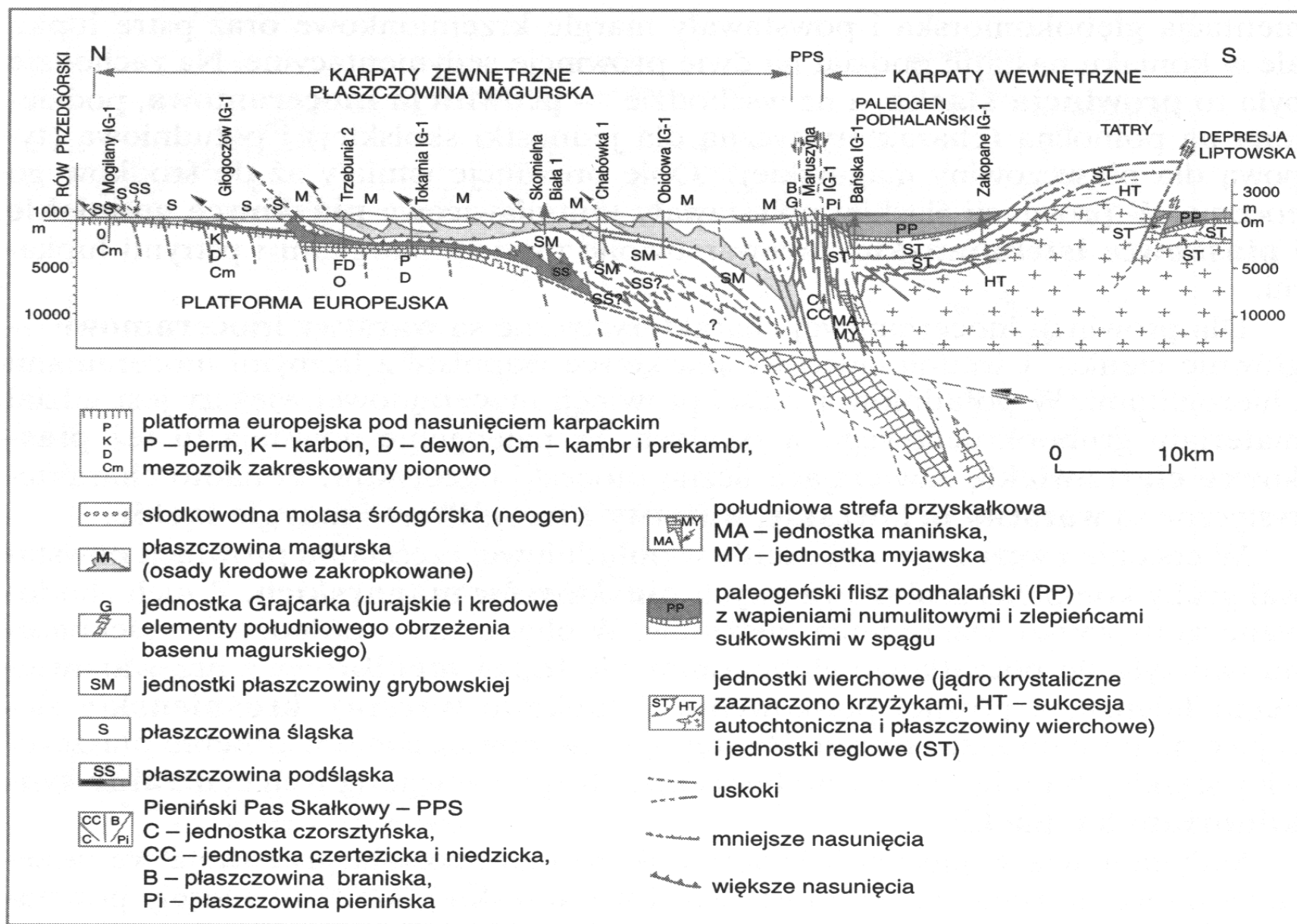
- - Przekrój geologiczny na linii Kraków–Zakopane (wg K. Birkenmajera, 1986 — uproszczony)
