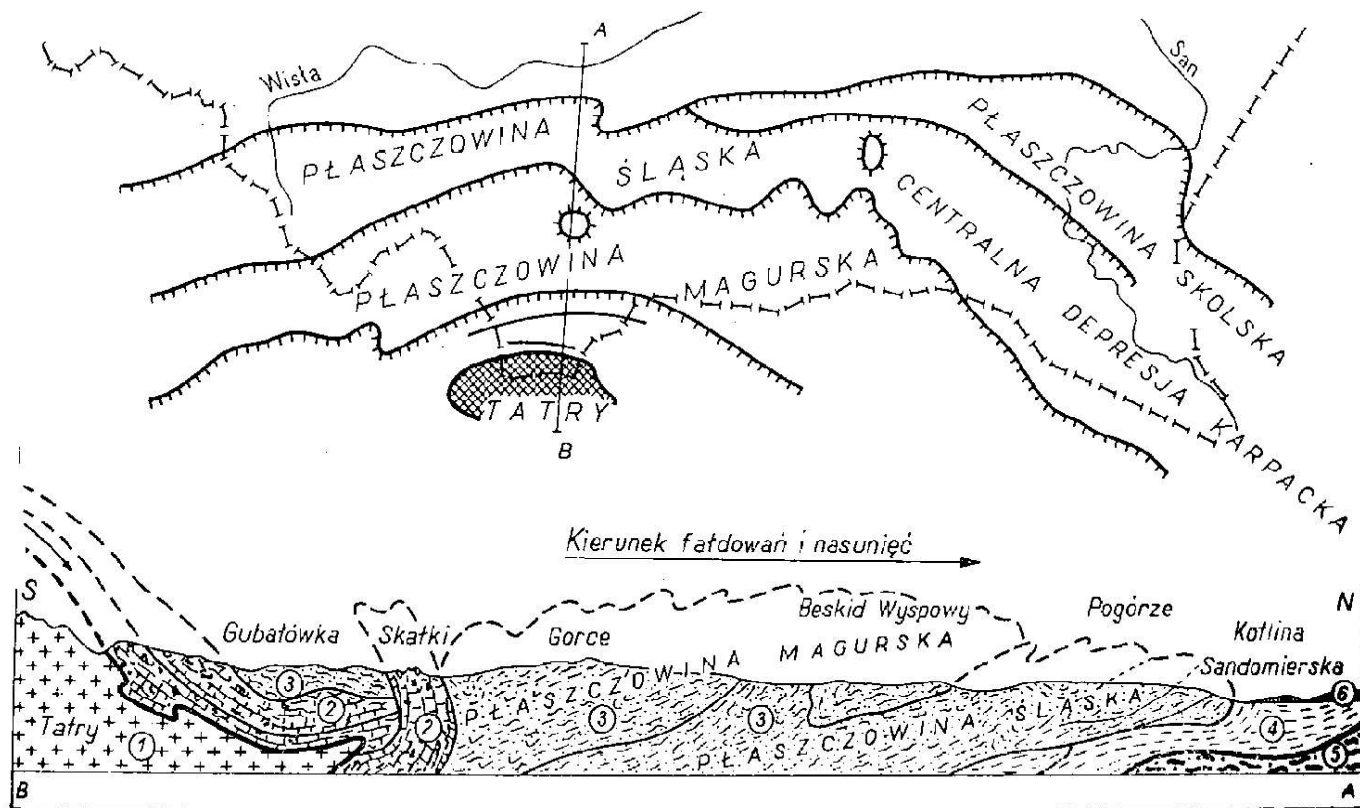
Ryc. 9. Zasięgi płaszczowin karpackich oraz schematyczny przekrój geologiczny przez Karpaty (wg K. Guzika)
